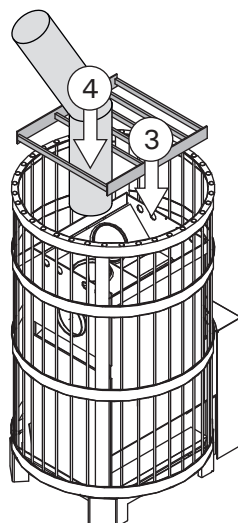
Figure 11. Connecting the stove to a masonry flue via the upper connection opening (all dimensions in millimeters) Obrázek 11. Připojení kamen ke komínu ve zdi skrz horní otvor (všechny rozměry jsou v milimetrech)
