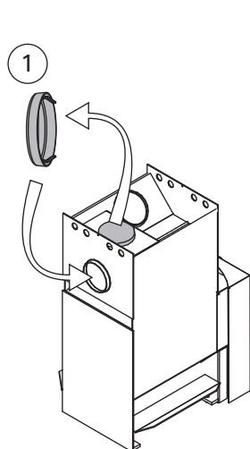
Figure 11. Connecting the stove to a masonry flue via the upper connection opening (all dimensions in millimeters) Obrázek 11. Připojení kamen ke komínu ve zdi skrz horní otvor (všechny rozměry jsou v milimetrech)
