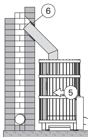
Figure 11. Connecting the stove to a masonry flue via the upper connection opening (all dimensions in millimeters) Obrázek 11. Připojení kamen ke komínu ve zdi skrz horní otvor (všechny rozměry jsou v milimetrech)
