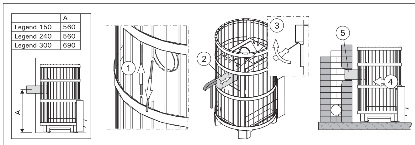
Figure 10. Connecting the stove to a masonry flue via the rear connection opening (A dimension in millimeters) Obr. 10 Připojení kamen ke komínu ve zdi skrz zadní otvor (všechny rozměry jsou v milimetrech)
