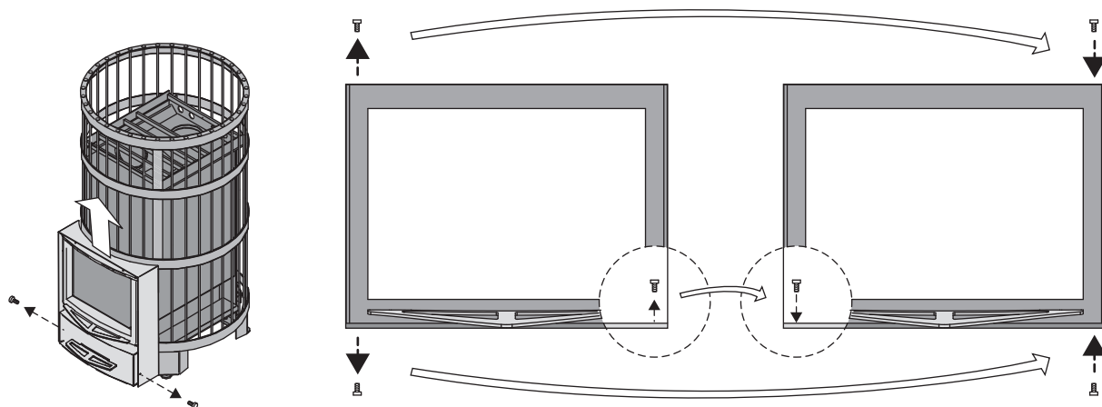
Figure 15. Changing the opening direction of the stove door Obr. 15. Změna směru otevírání dvířek kamen
