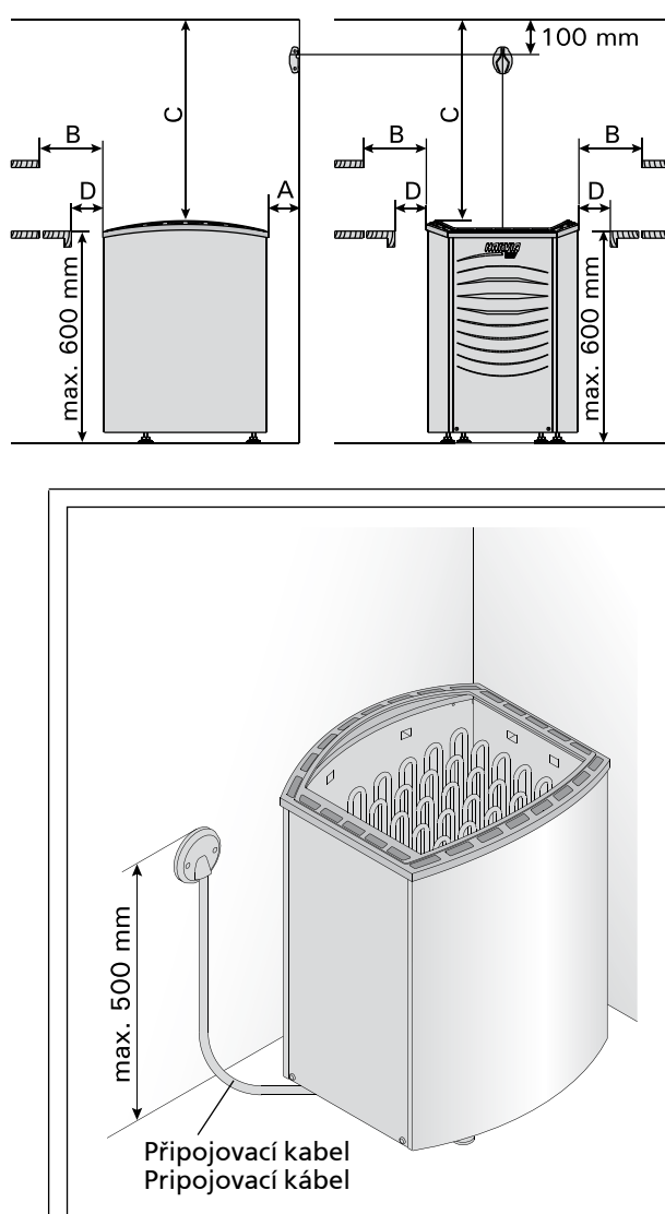
Obrázek 4. Zapojení topného tělesa Obrázok 4. Prípojka saunových kachiel'
