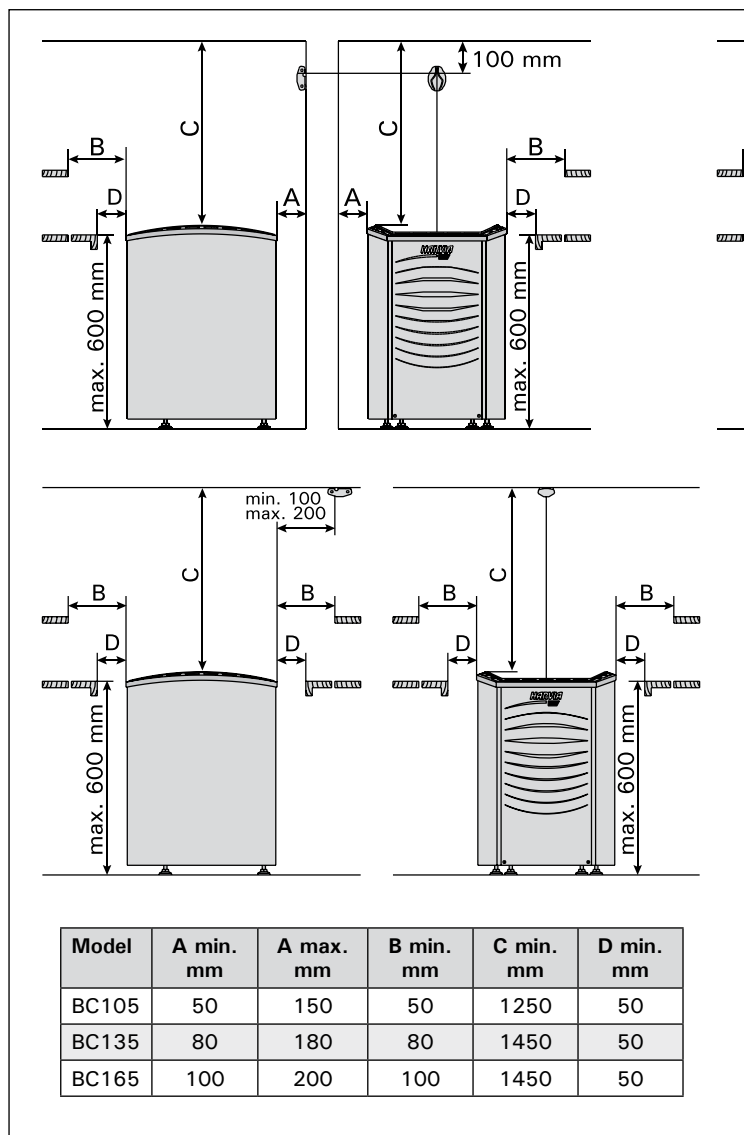
Obrázek 3. Bezpečné vzdálenosti pro topné těleso Obrázok 3. Bezpečné minimálne vzdialenosti saunových kachiel'
